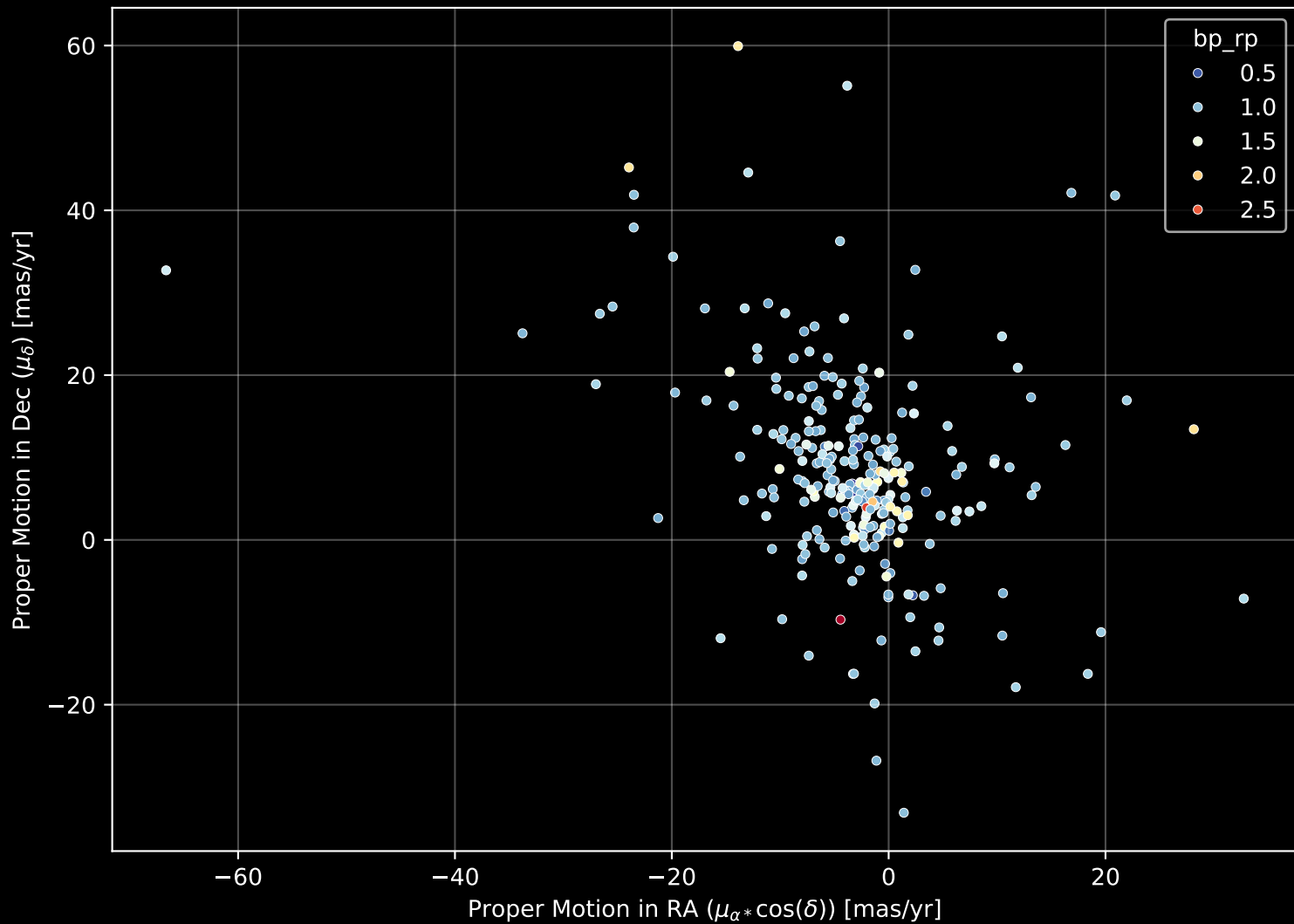
GALAH DR4 Field: [2176] Proper Motion Diagram (n= 271)
