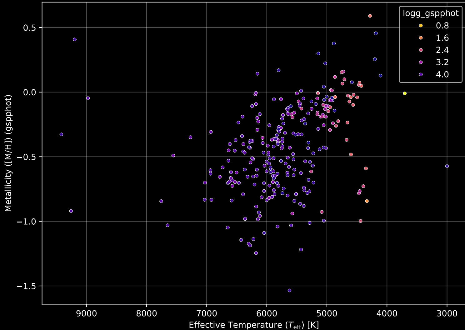
GALAH DR4 Field: [2176] Stellar Population Parameters (n= 271)
