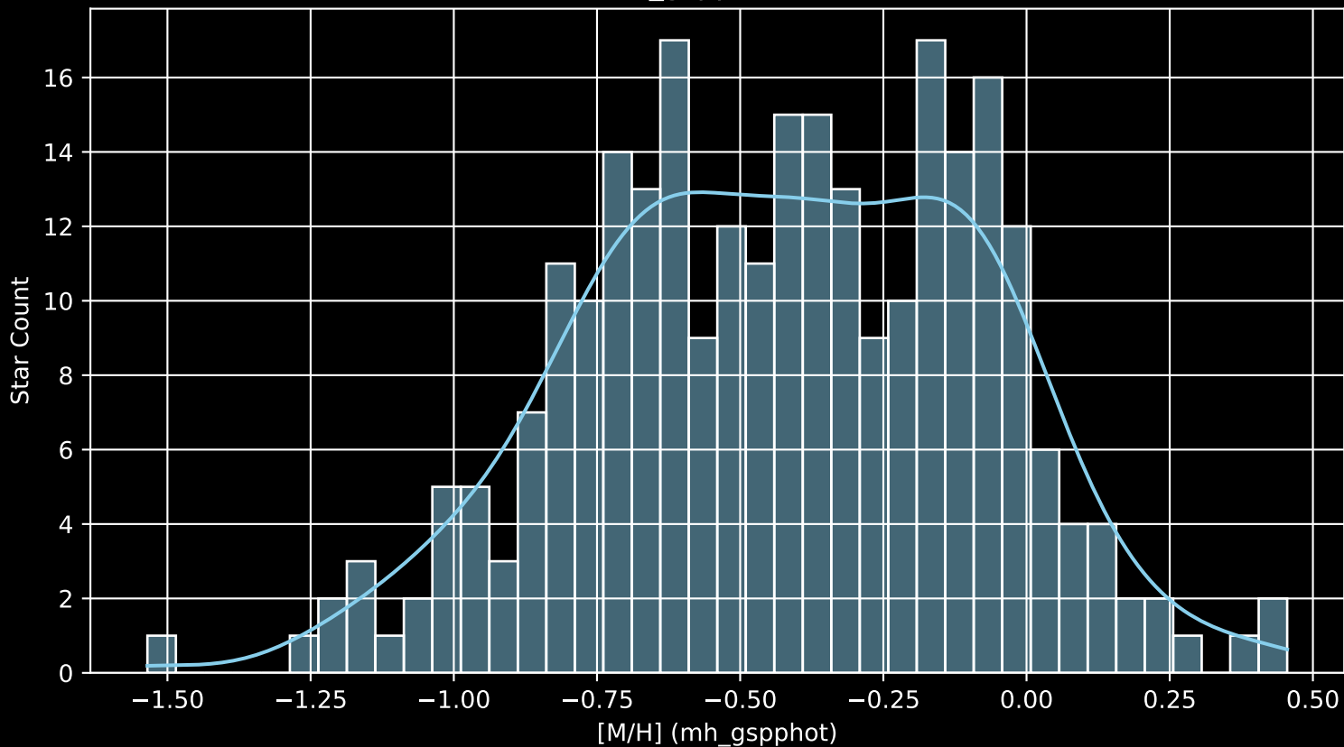
GALAH DR4 Field: [2176] [M/H] (mh_gspphot) (n= 270)
