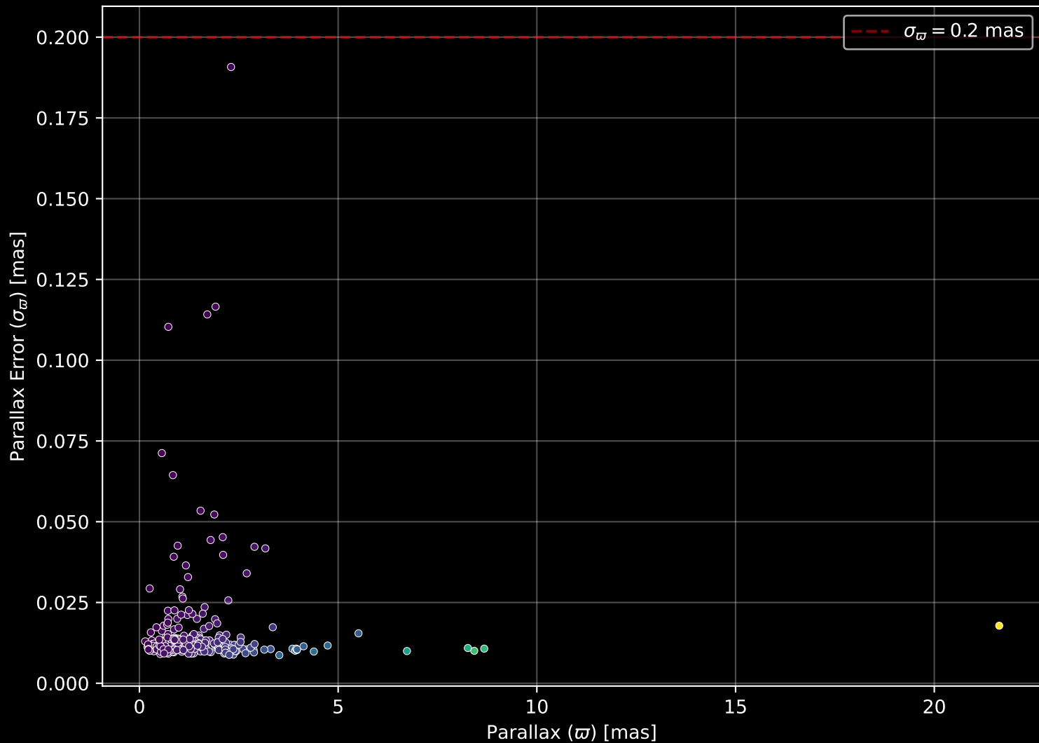
GALAH DR4 Field: [2176] Parallax Quality (n= 271)
